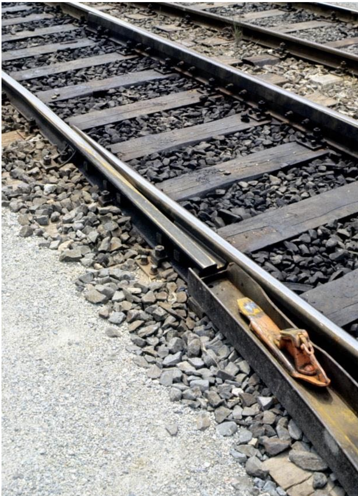
Hemmschuh-Auswurfbremse, Wr.Neustadt, 26.7.1986
